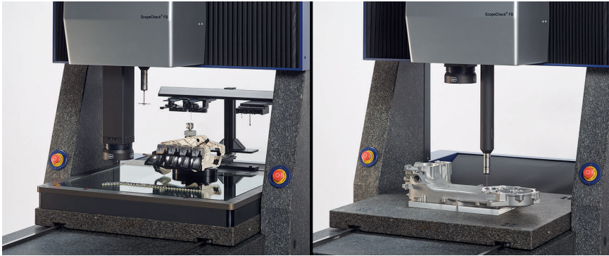
Bild 2. Das kompakte Portalgerät ermöglicht Multisensor-Messungen ohne Messbereichseinschränkungen durch die jeweils nicht genutzte Sensorik (links), schwere Werkstücke können direkt auf dem Mess-tisch gemessen werden (rechts). (© Werth)
