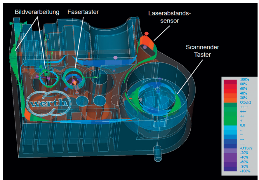
Bild 1. Multisensor-Messung: Der Bildverarbeitungssensor ermöglicht eine schnelle Kantenmessung, kleine Bohrungen sind für den taktil-optischen Mikrotaster problemlos zugänglich. Mit dem Laserabstansensor kann ein schnelles Scanning in der Ebene durchgeführt, mit einem Taster auch der senkrechte Zylinder gemessen werden. (© Werth)
