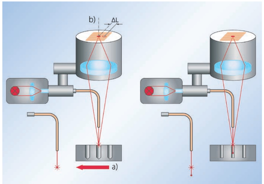
Bild 1. Funktionsprinzip des Fasertasters: Einkugeltaster (links): Die Bewegung des Messobjekts (a) führt zur Antastung und Auslenkung \Delta L vom Sensornullpunkt in der Bildebene der Kamera (b). Zweikugeltaster (rechts): Auch beim Antasten in größerer Tiefe erfolgt keine Abschattung der Kugel durch das Objekt.
