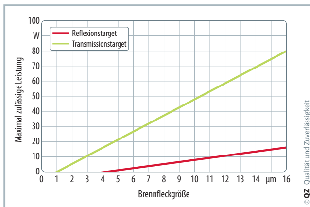
Bild 1. Maximal zulässige Leistung in Abhängigkeit von der angestrebten Auflösung (Brennfleckgröße) für Röhren mit Transmissions- (grün) bzw. Reflexionstarget (rot) für den in der Koordinatenmesstechnik wichtigen Bereich (© Werth)
